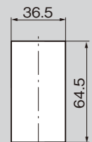
パネル穴明け寸法 Panel drilling dimensions
