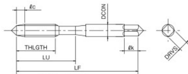
新形状 New Dimension
