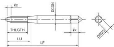
旧形状 Old Dimension
