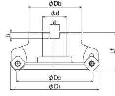
Type2 油穴なし Without coolant hole
