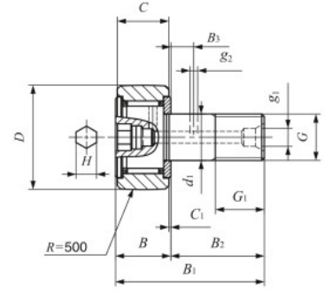
CF...BR Stud dia d_1 12-30mm
