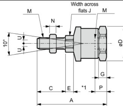
Rod nut dimensions
