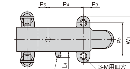
C-1157-1-A (平行取付けタイプ) (Parallel installation type)
