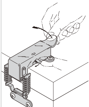
Bタイプ B-type
