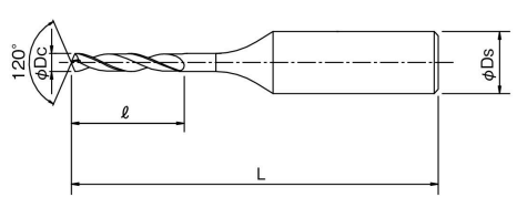
フォーファセットポイント Four Facet point (Dc ≤ 1.15mm)
