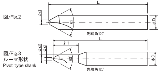
図/Fig.2 : φD 最大面取り径 Max. Chamfering Dia. 図/Fig.3 : φd1 最大面取り径 Max. Chamfering Dia. 図/Fig.2,3 : φd 最小面取り径 Min. Chamfering Dia.
