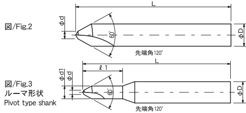
図/Fig.2 : φD 最大面取り径 Max. Chamfering Dia. 図/Fig.3 : φd1 最大面取り径 Max. Chamfering Dia. 図/Fig.2,3 : φd 最小面取り径 Min. Chamfering Dia.
