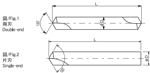
図/Fig.1, 2 : \phi D 最大面取り径 Max. Chamfering Dia.
